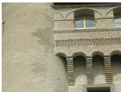
Assainissement des briques dégradées et conservation des briques encore saines
