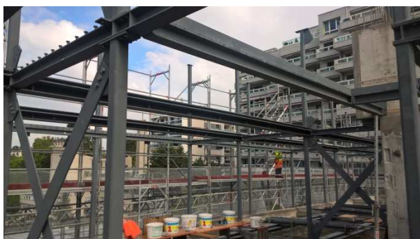
Montage de la charpente
