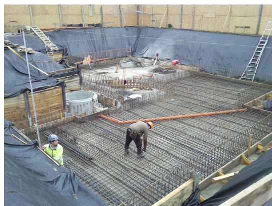
Ferraillage du radier.
