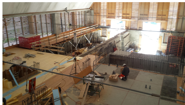
Réalisation de nouvelles dalles (2 niveaux) dans le volume existant après mise en place de tirants provisoires. La dalle du niveau 2 fera office de tirant pour la charpente existante.
