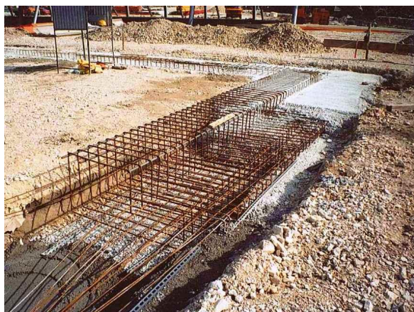
Bétonnage des fondations
