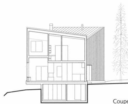
Coupe
